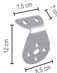
Staffa Parete / Soffitto 6000 INOX
