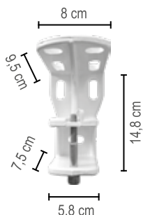
Mensola P/S 8000 C
