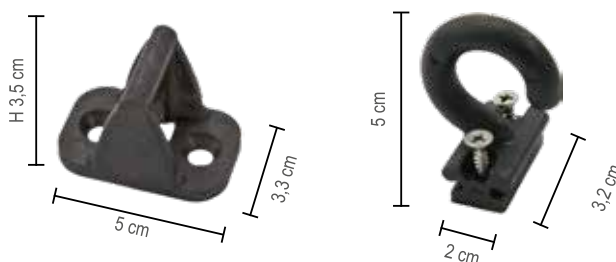
Attacco a Pavimento Roma a richiesta
