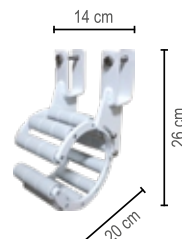
Reggirullo Rodi
