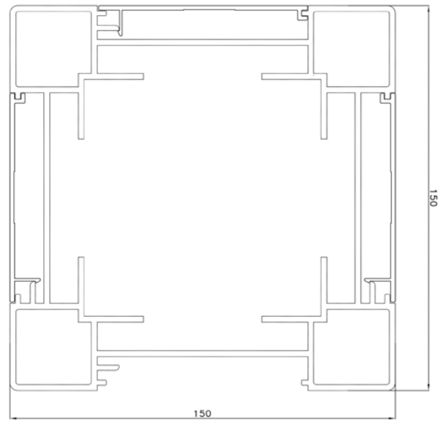
Piede Bioclimatica
