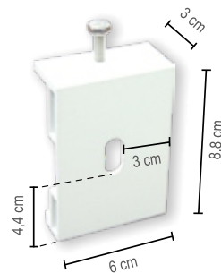
Staffa a Soffitto Tende cassonate a caduta
