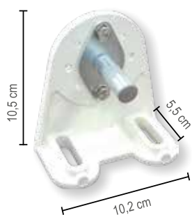
Staffa
