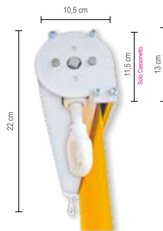
Cassonetto 4000 R
