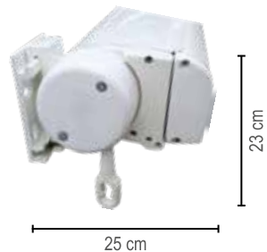
Ingombro Newbox
