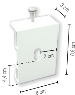
Staffa a Soffitto mod. 4000
