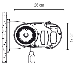
Cassonetto
