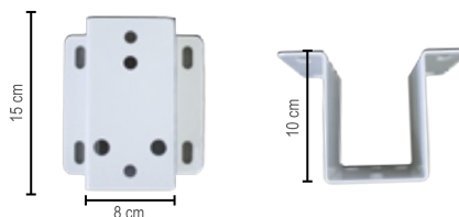
Distanziale opzionale a richiesta € 30,00 cad.
