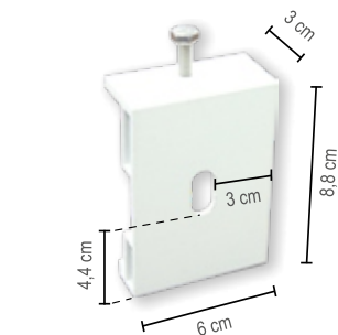
Staffa a Soffitto mod. 4000
