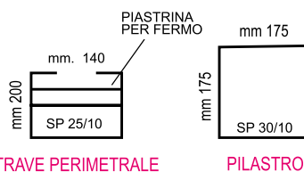
TRAVE PERIMETRALE
