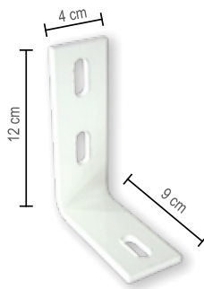
Staffa a Parete Tenda a caduta cassonata
