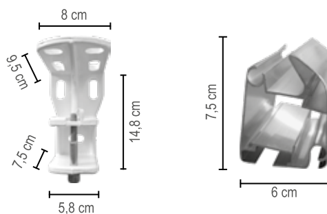
Mensola P/S 8000 C
