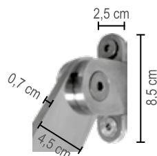
Attacco Braccio a muro Tenda 6000 INOX
