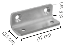
Staffa a vano braccio 6000 INOX
