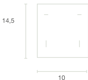
Staffa a muro
