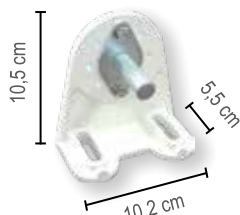
Staffa Parete / Soffitto Tenda 6000
