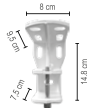
Mensola P/S 9000K17 IN
