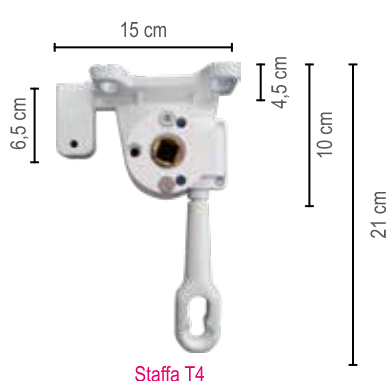
Staffa T4
