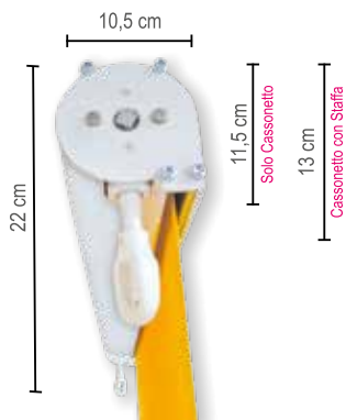
Cassonetto 7000 R
