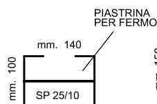
TRAVE PERIMETRALE
