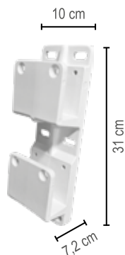
Staffa a Parete 8000 G
