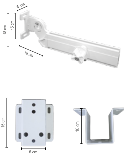
Distanziale opzionale a richiesta € 35,00 cad.
