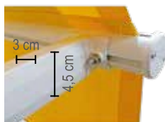
Braccetto 6000 con attacco al Terminale
